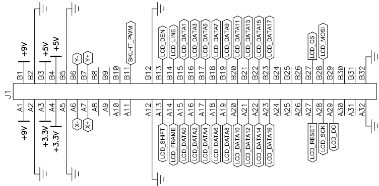
Display Connector V1
