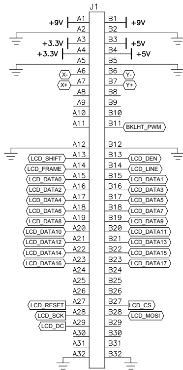
Display Connector V1
